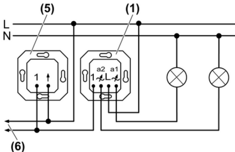
Afbeelding 3: Aansluitschema
